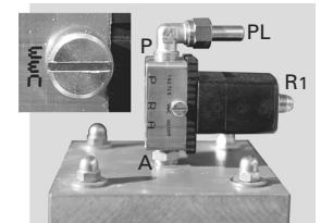
Śruba szczelina Pozycja «płukanie wsteczne»
