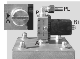
Vite a intaglio Posizione «controlavaggio»
